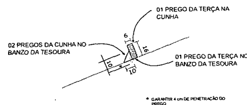
2 TERÇAS - DETALHES SEM ESCALA
