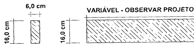
1 TERÇAS - BITOLA SEM ESCALA
