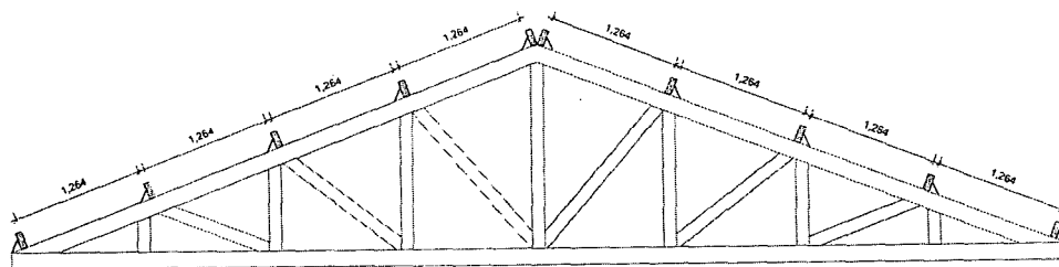
3 TERÇAS - MONTAGEM - PALANQUE SEM ESCALA
